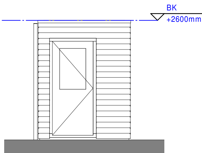
Rechter zijaanzicht
